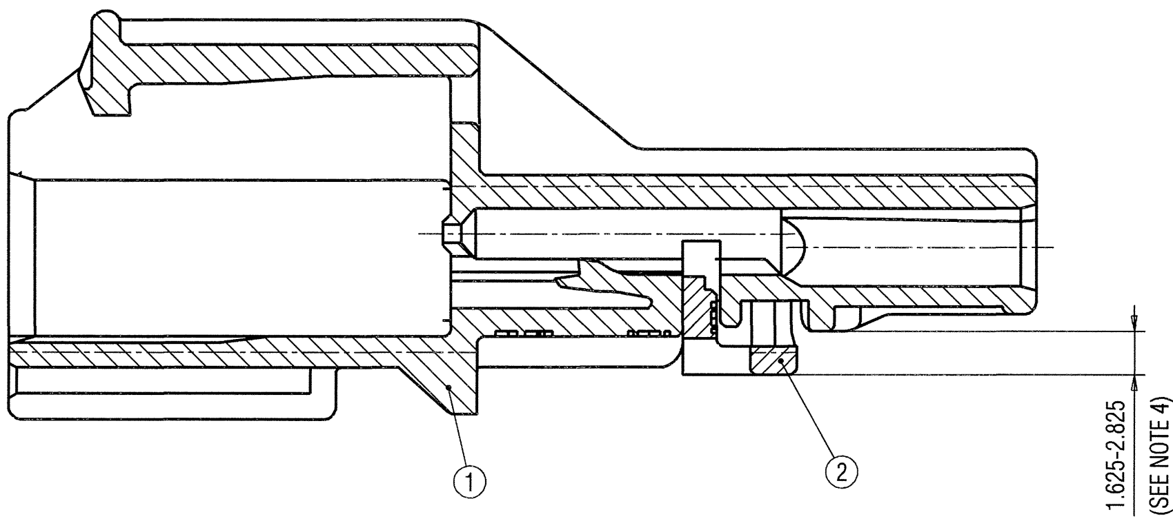
SECTION A-A
